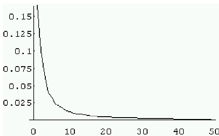
FIGURE 2. — \lambda_2(p_j) pour j \geq 2 .
