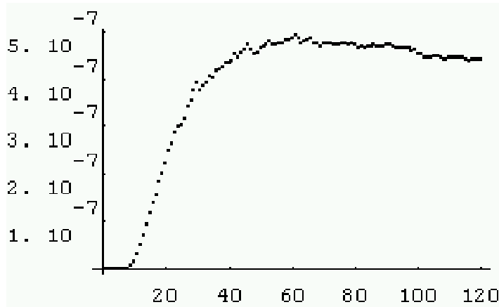
FIGURE 1.— \lambda_9(p_j) pour 1 \leq j \leq 120 .
